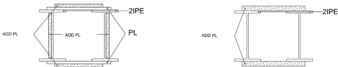
شکل (۲-۴۱): نمایی از جزئیات چند نمونه تقویت ستون
